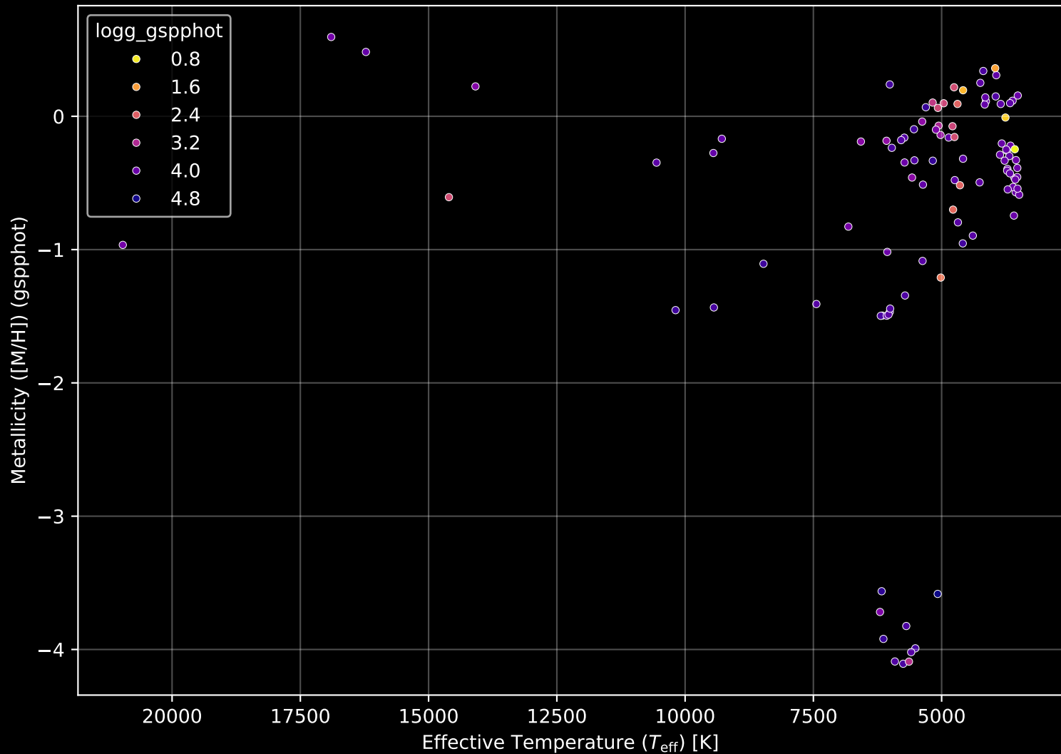
APOGEE DR17 Field: [ORIONA-B] Stellar Population Parameters (n= 102)
